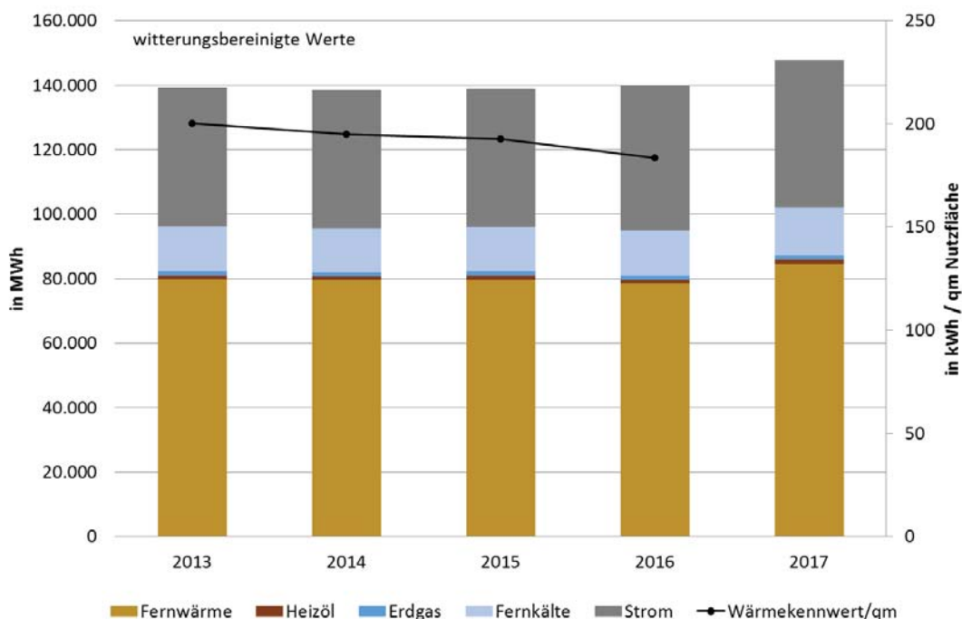
Abbildung 7: Entwicklung des Energieverbrauchs der Universität Heidelberg 2013 bis 2017 (witterungsbereinigt)
