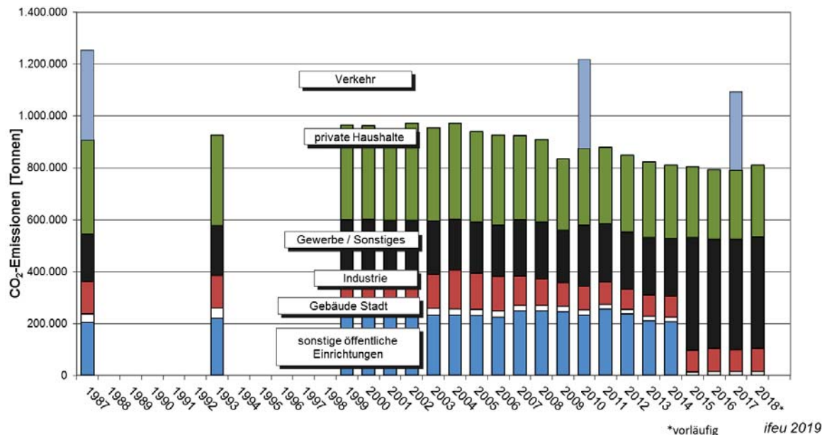
Abbildung 1: Entwicklung der stationären Endenergie in Heidelberg von 1987 bis 2018 nach Sektoren
