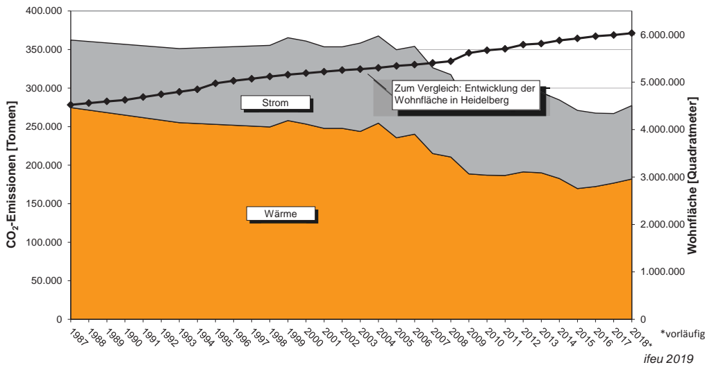
Abbildung 6: CO 2 -Emissionen der privaten Haushalte in Heidelberg 1987 bis 2018 nach Wärme und Strom (witterungskorrigierte Darstellung)
