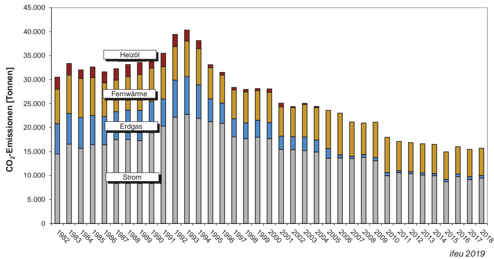
Abbildung 8: Entwicklung der CO 2 -Emissionen der Gebäude der Stadt Heidelberg (witterungskorrigierte Darstellung) *ab 2006 werden Erdgasverbräuche teilweise über die Wärmelieferung bilanziert, deshalb sind die Emissionen durch Erdgas in der Fernwärme enthalten.
