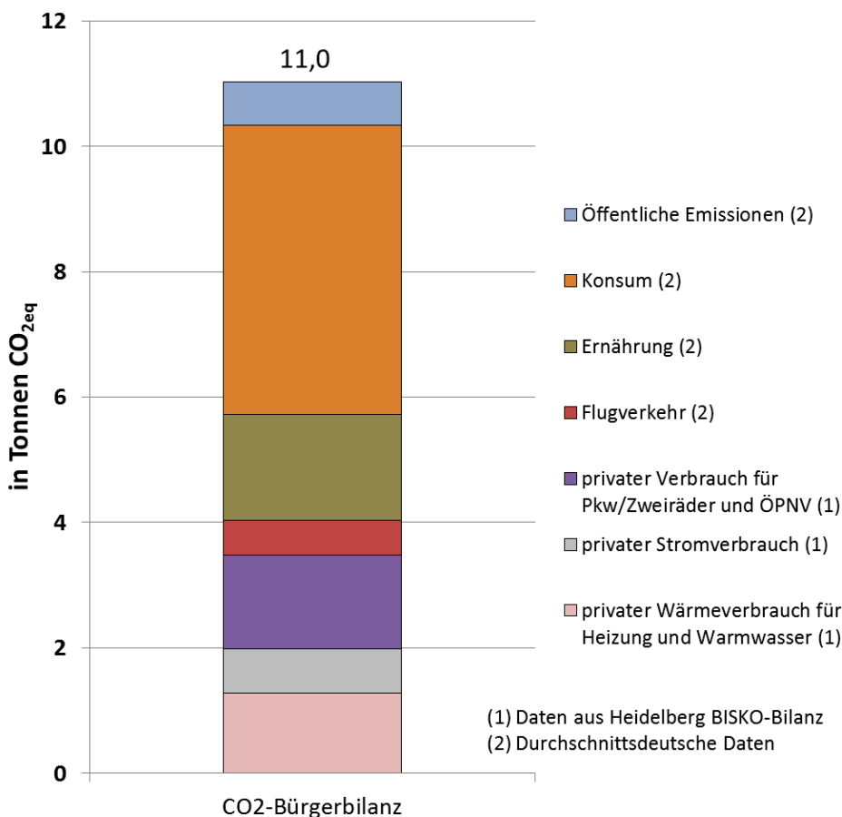
Abbildung 14: CO 2 -Bürgerbilanz mit lokalen und deutschlandweiten Daten
